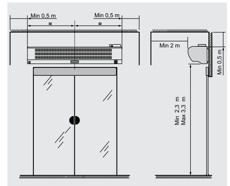
Montaj ölçüleri
